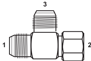
F6602 FO-FJS-FO TEE
